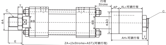
外形尺寸表 Dimension table
