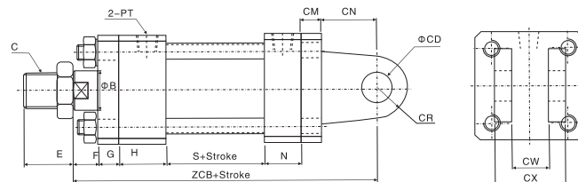
外形尺寸表 Dimension table
