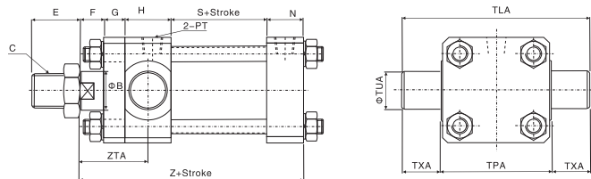
外形尺寸表 Dimension table
