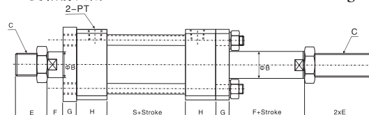
外形尺寸表 Dimension table
