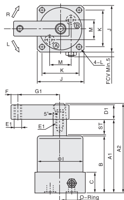
外形尺寸表 Dimension table
