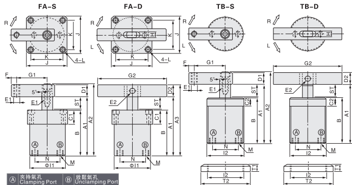
外形尺寸表 Dimension table
