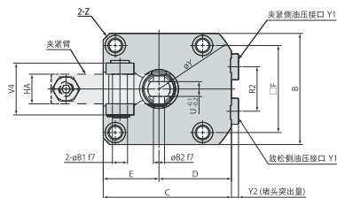
外形尺寸图 (夹緊检测型)
